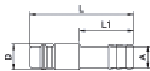
Stem
